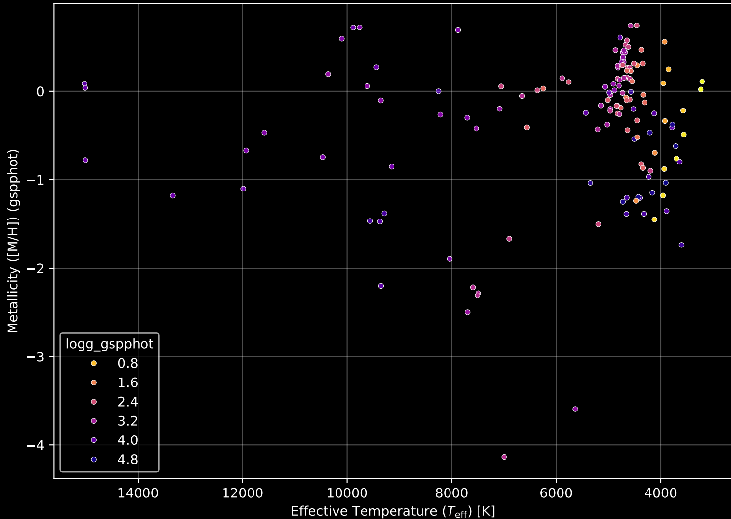
APOGEE DR17 Field: [010+00] Stellar Population Parameters (n= 141)
